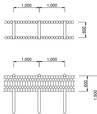
D-0011 スタンド土留
