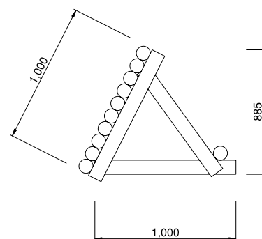
D-0005 根固工
