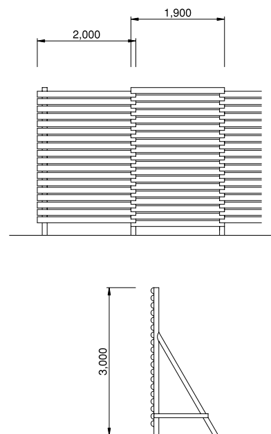
D-0008 防風柵
