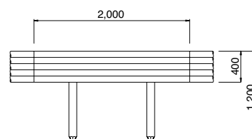
D-0012 木製ふとんかご
