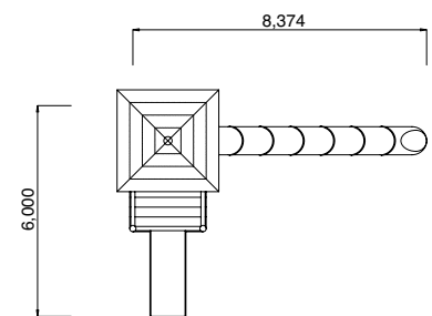
Y-0005 コンビネーション遊具
