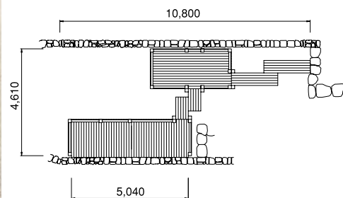
SD-0014 デッキ
