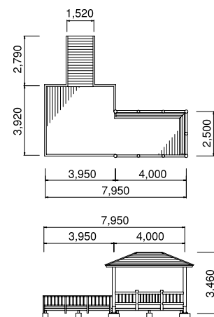
SD-0014 デッキ
