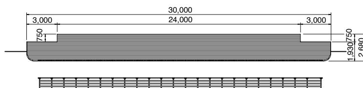
SD-0020 デッキ
